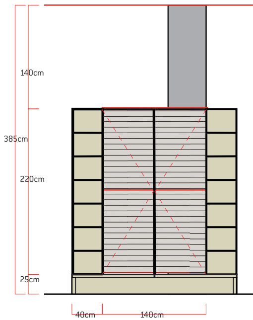
aanzicht korte zijde vanaf Feduzzipteintje
