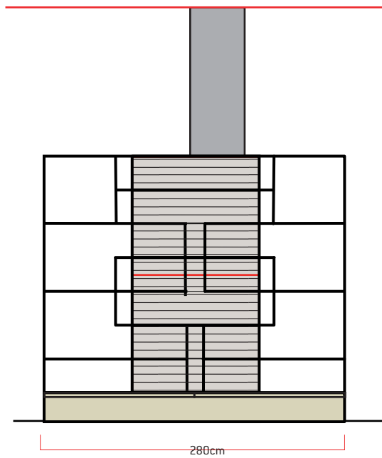
aanzicht lange zijde
