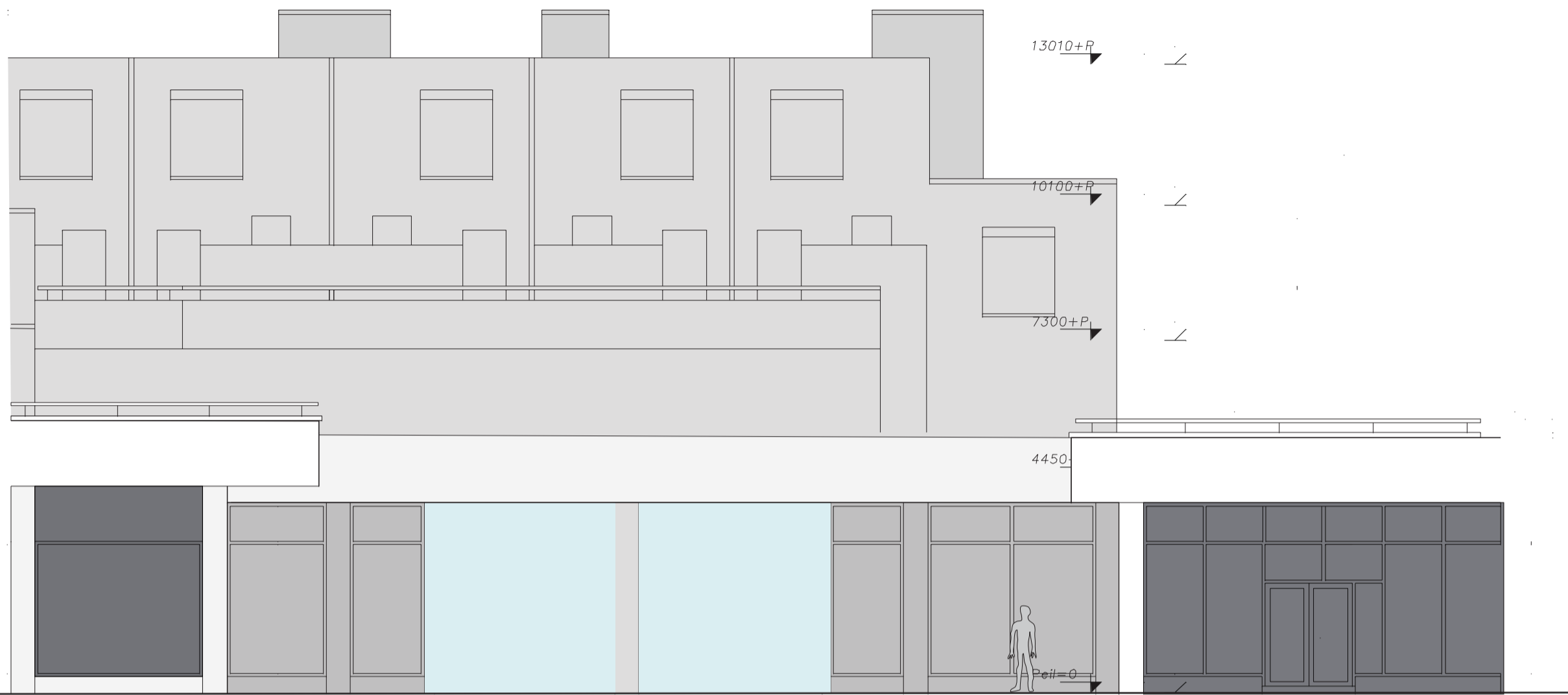
AANZICHT GEVEL / ONDERDOORGANG VANAF DE NIEUWE WETERINGSTRAAT
