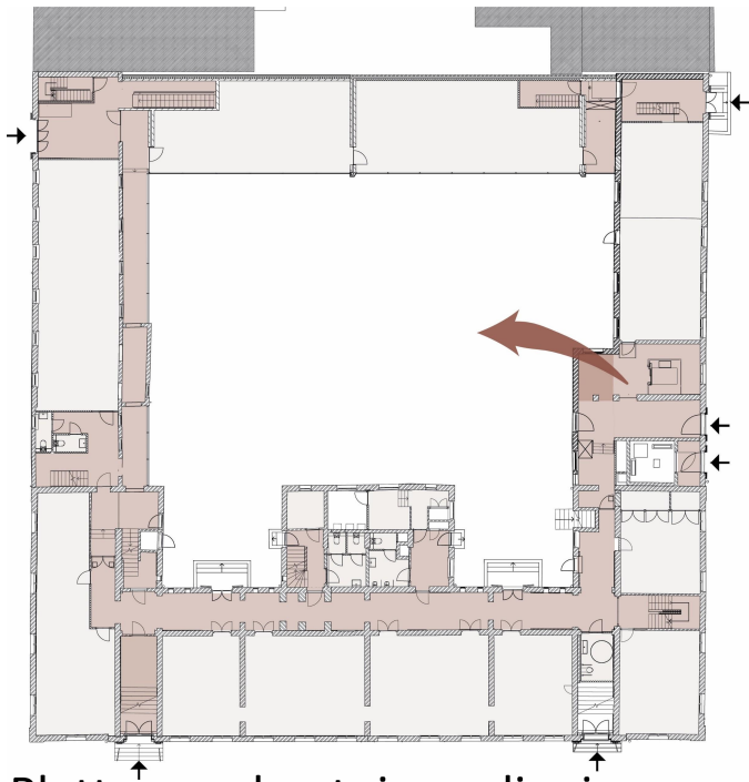
Plattegronden tuinverdieping
